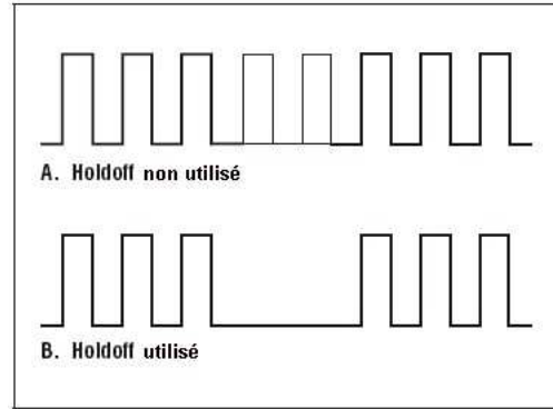
Figure 3. Utilisation du contrôle HOLD OFF.
